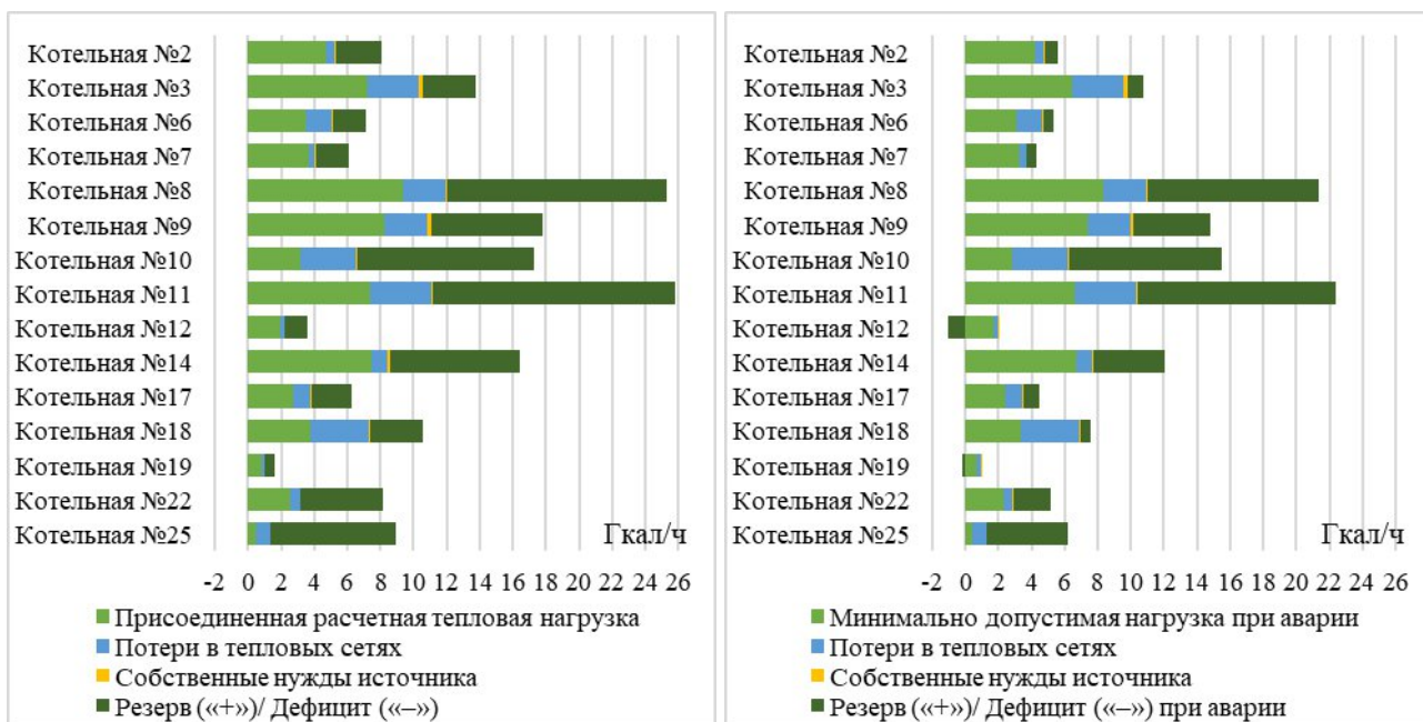
Рисунок 3.9. Баланс мощности источников в штатном и аварийном режимах
