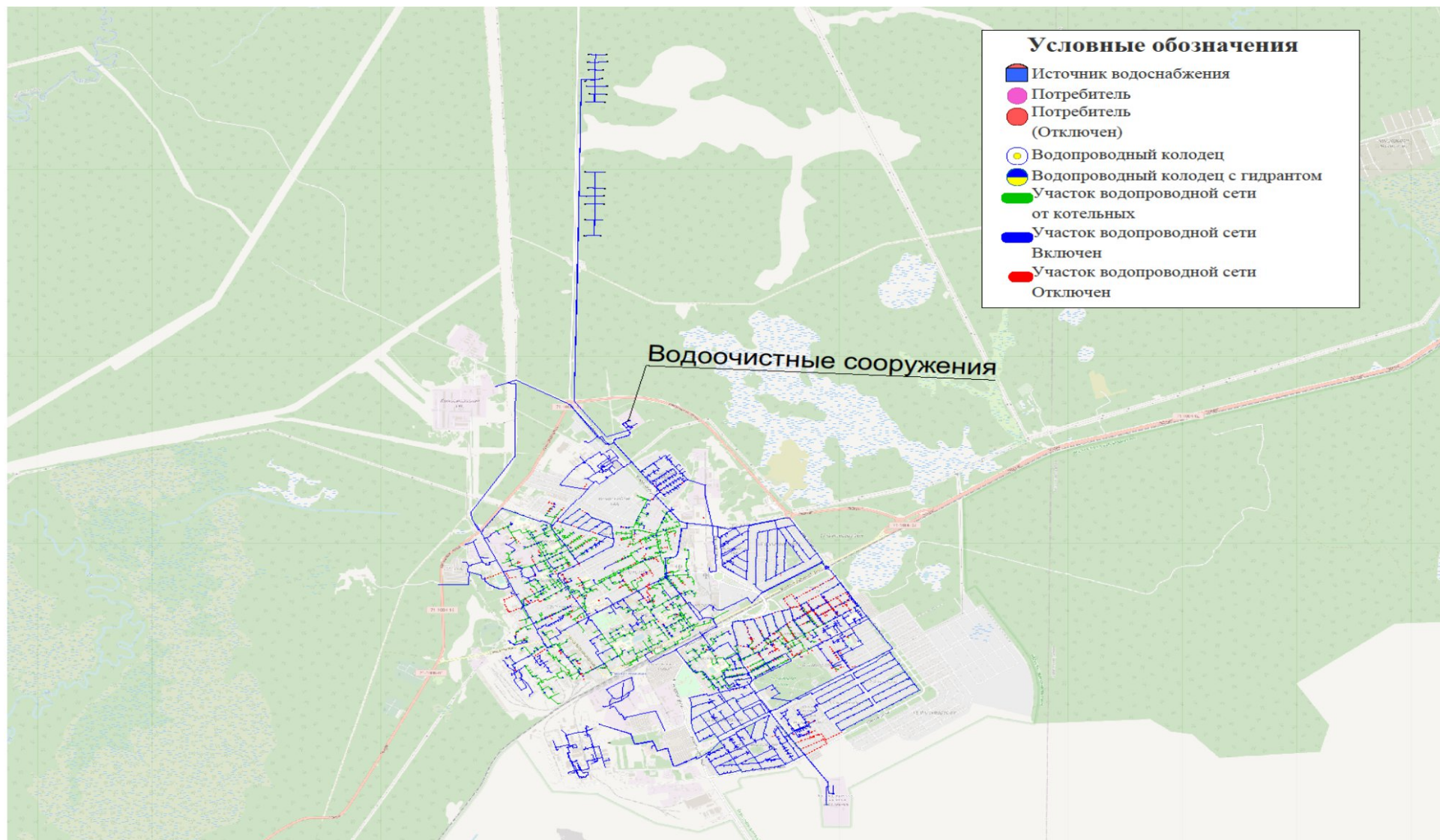
Рисунок 3.12. Схема сетей водоснабжения г. Югорска
